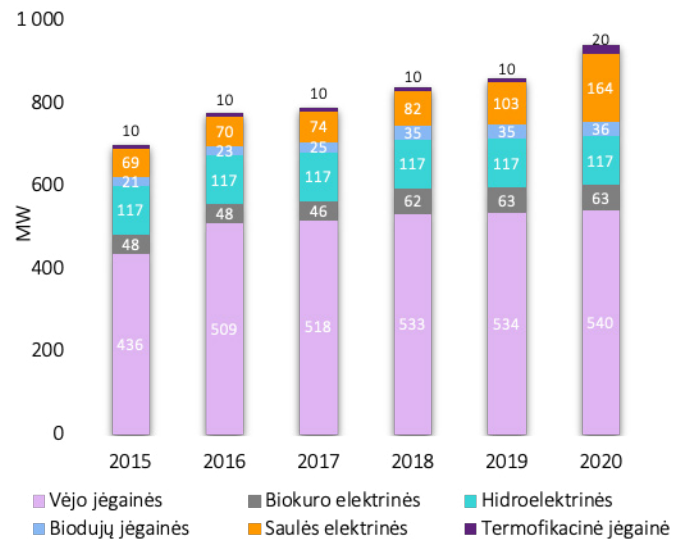
9 pav. Elektros energijos gamybos įrenginių galia 2015-2020 m. Duomenų šaltinis: Lietuvos statistikos departamentas
