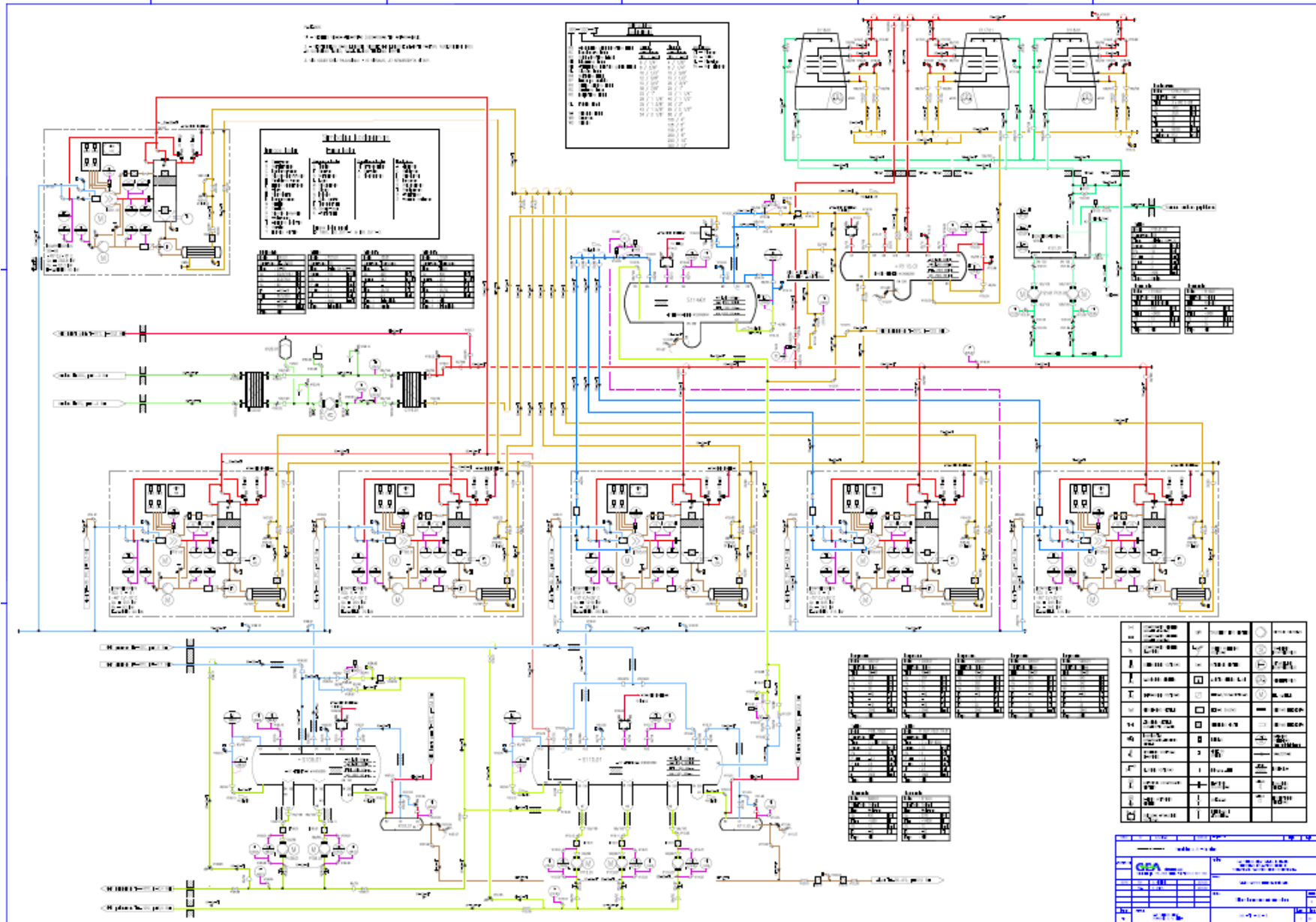
Schema 1: BIOVELA-UTENOS MĒSA, UAB šalčio gamybos technologinė dalis
