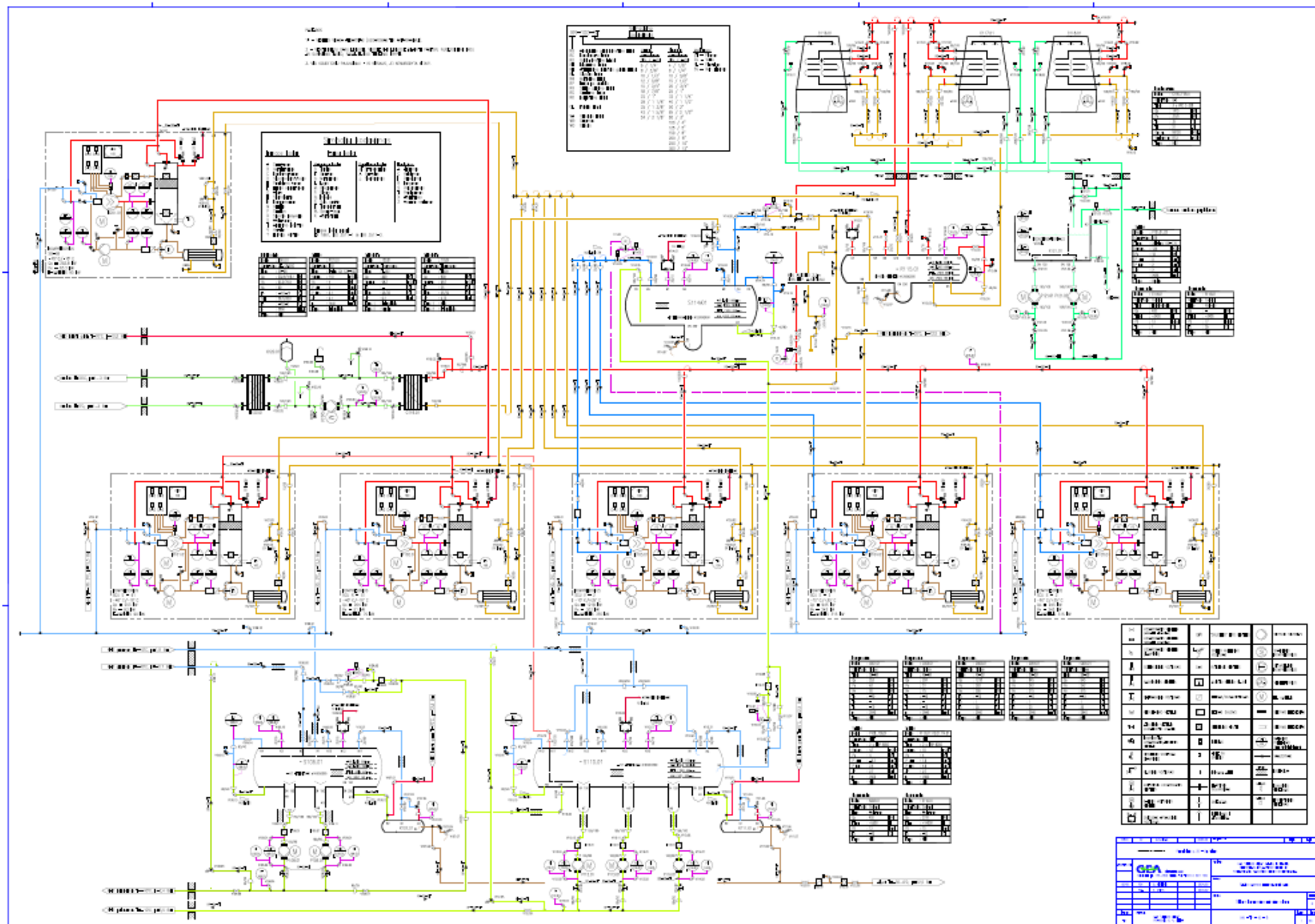
Schema 1: BIOVELA-UTENOS MĖSA, UAB šalčio gamybos technologinė dalis
