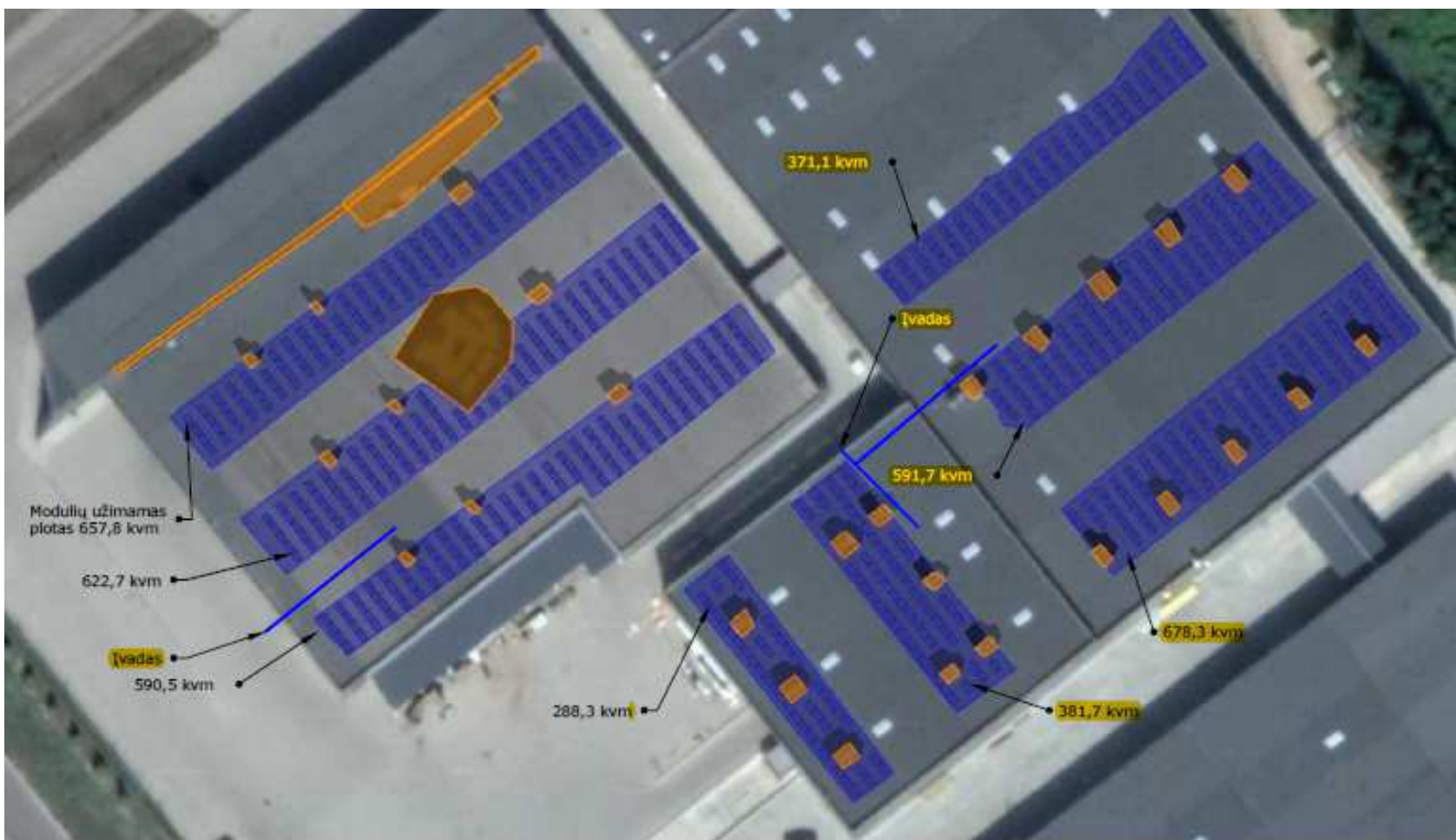
Fotomodulių išdėstymas ant pastato stogo, Industrijos g.5, Biruliškės, Kauno r., planas
